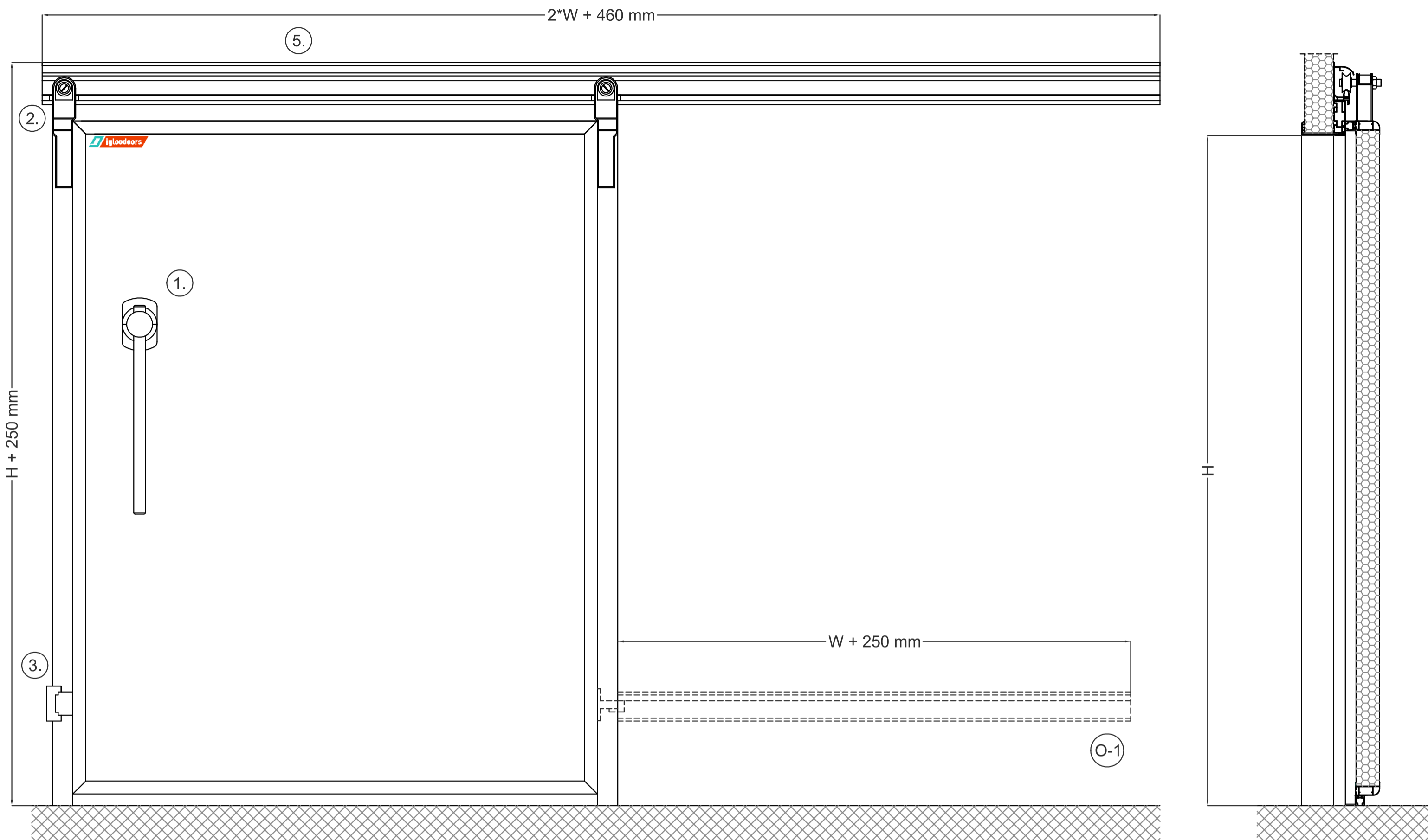
"A" metszet M1:4
