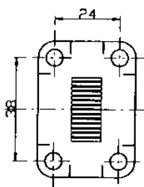
Piastrina per la regolazione verticale Vertical adjustment plate
